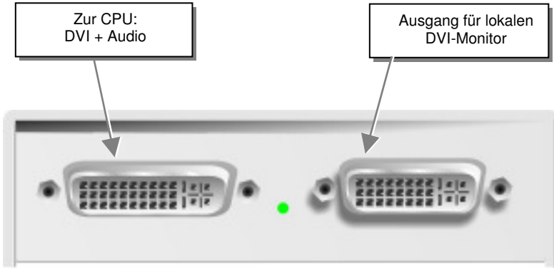
DVXi/ME Media-Extender Typ K466-AM, K466-AS, K467-AM, K467-AS, 468-AM und K468-AS Local Unit
