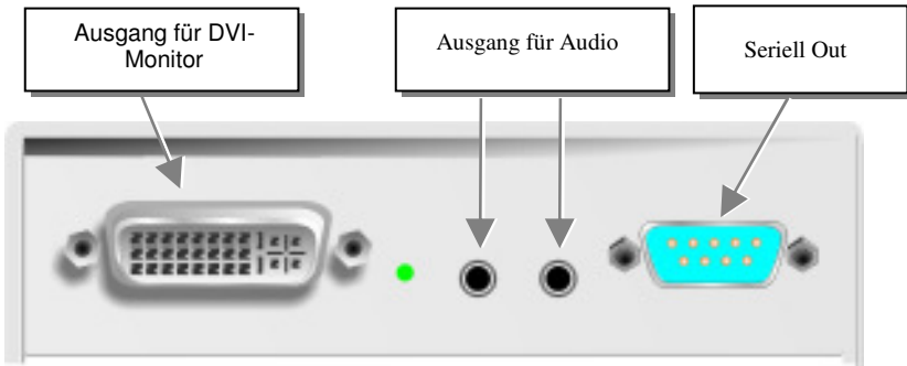
DVXi/ME Media-Extender Typ K466-AM, K466-AS, K467-AM, K467-AS, 468-AM und K468-AS Remote Unit
