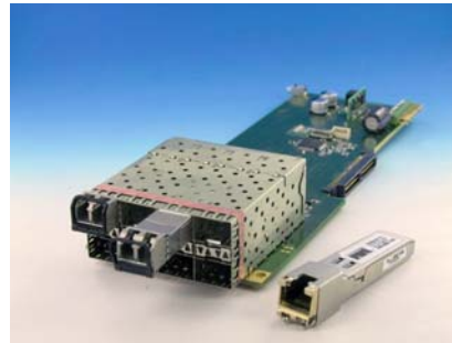
Glasfaser E/A Baugruppe
